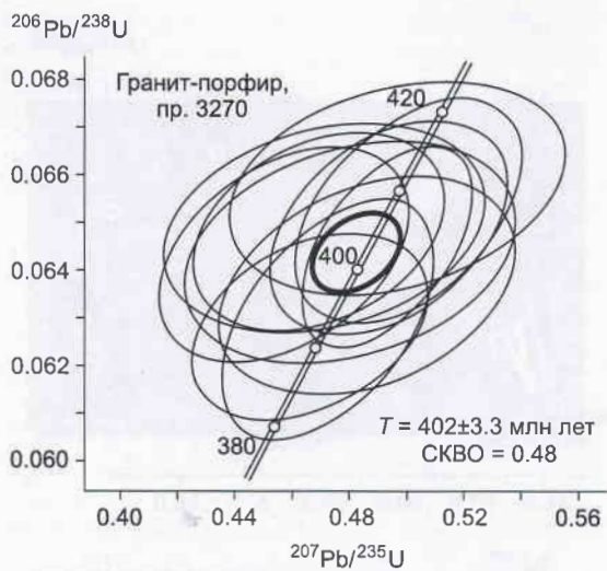
Рис. 2. U-Pb диаграммы и морфологические особенности цирконов из кембрийских (а), силурийских (б) и раннедевонских (в) гранитоидов Батеневского кряжа.
