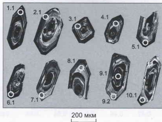
Рис. 2. U-Pb диаграммы и морфологические особенности цирконов из кембрийских (а), силурийских (б) и раннедевонских (в) гранитоидов Батеневского кряжа.
