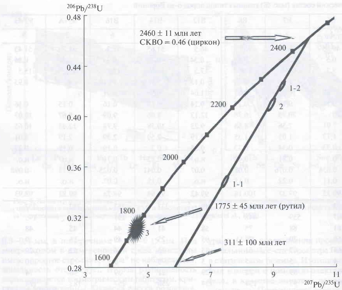
Рис. 5. U-Pb диаграмма с конкордией для циркона и рутила из габбронорит-анортзита (обр. 99VG).
