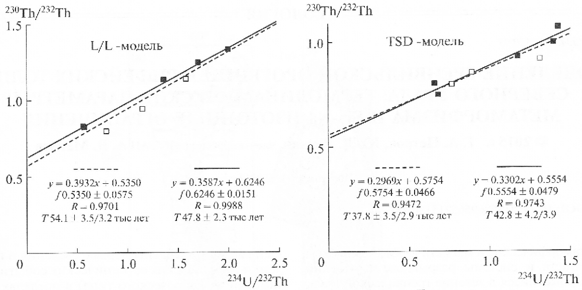
Рис. 2. Изохроны, построенные по образцам органогенных отложений из разреза Курьятор. Прерывистые линии — изохроны по всем 8 проанализированным образцам, сплошные линии — изохроны по 5 выбранным образцам (темные квадраты).
