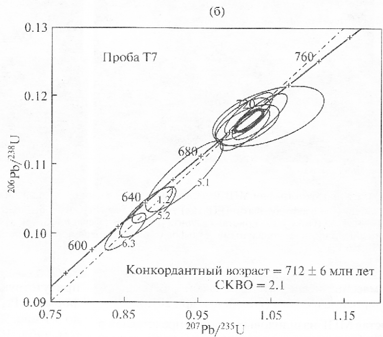
Фиг. 17. Морфология зерен циркона из меланогаббро Тартайского массива с участками изотопных исследований (а) и U-Pb-геохронологические данные (SIMS) (б).
