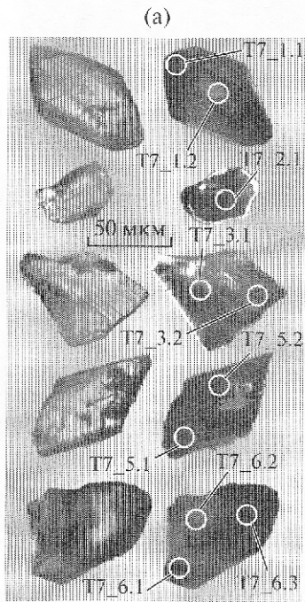
Фиг. 17. Морфология зерен циркона из меланогаббро Тартайского массива с участками изотопных исследований (а) и U-Pb-геохронологические данные (SIMS) (б).
