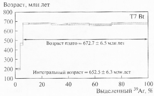
Фиг. 18. Ar-Ar-возрастные спектры биотита для Тартайского массива.
