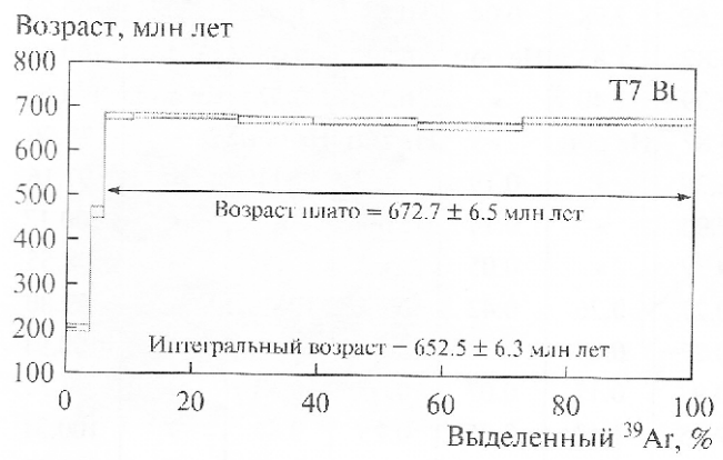
Фиг. 18. Ar-Ar-возрастные спектры биотита для Гар-тайского массива.
